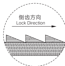
电线固定部(锁紧帽)
