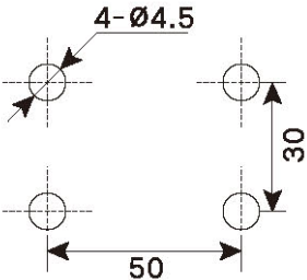
露出表面安装用支架 注：配件：M4-15螺丝/螺母/弹簧 各4枚(购买支架时提供)
